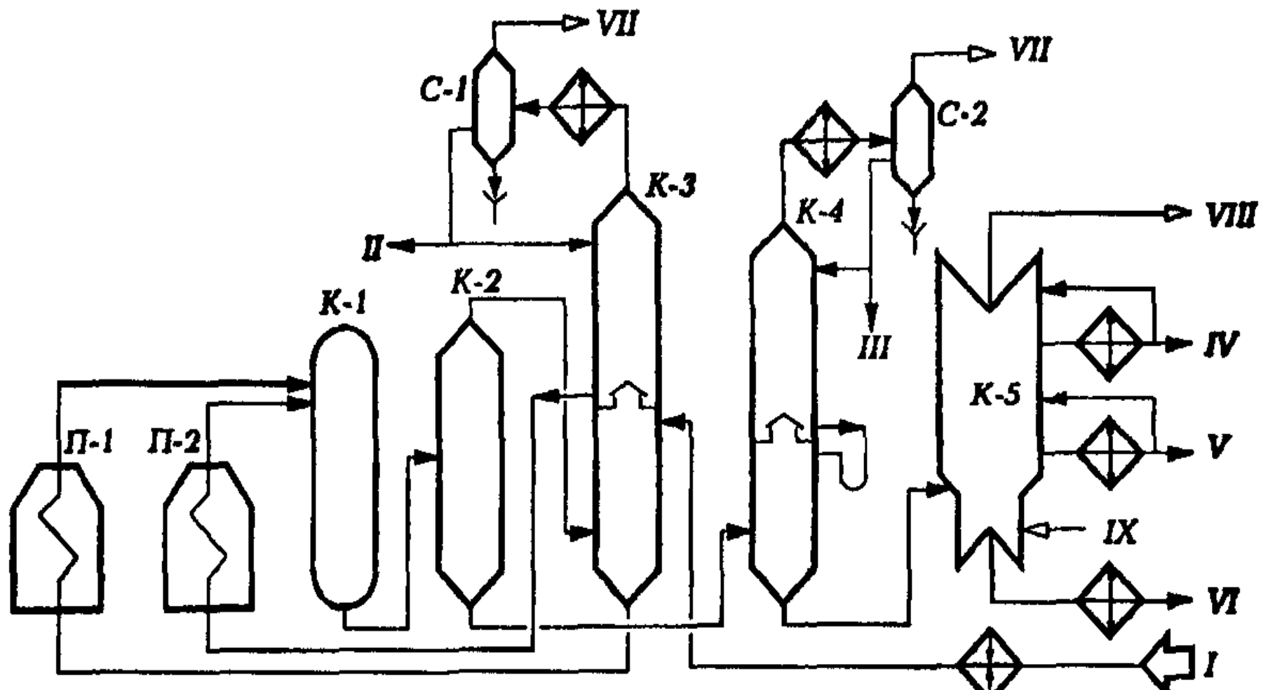
Сурет 1. Дистиллятты шикізатты термиялық крекингтеу қондырғысының принципиалдық технологиялық сызба-нұсқасы.
